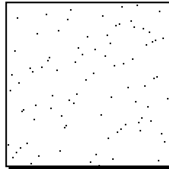
Linear Shuffle 2
